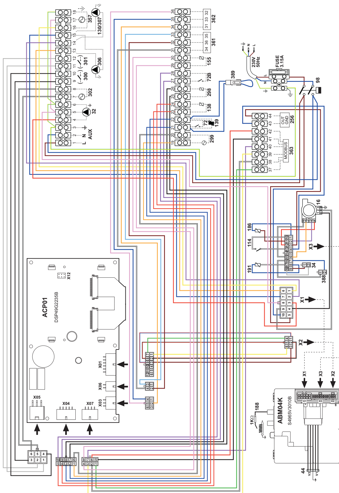
рис. 99- Электрическая схема моделей TORO W 60 и TORO W 80
