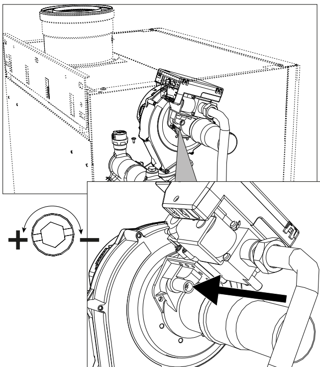
fig. 76- Réglage maximum modèles W 60 et W 80
