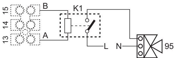
рис. 96- Подключение 3-х ходового клапана с 2 проводами
