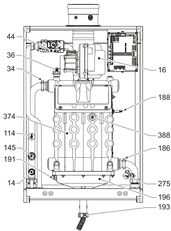
рис. 90- Общий вид, мод. TORO W 99 и TORO W 120
