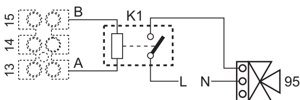
fig. 96- Conexión de la válvula de 3 vías con 2 hilos
