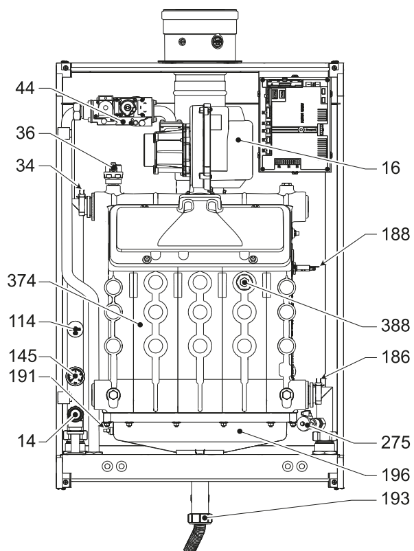
рис. 91- Общий вид, мод. TORO W 150
