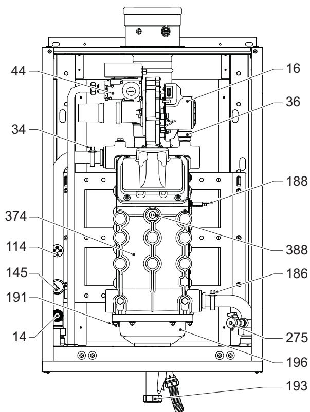
fig. 89 - Vista generale mod. TORO W 60 e TORO W 80
