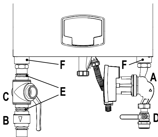
fig. 34- Chaudière avec les kits installés
