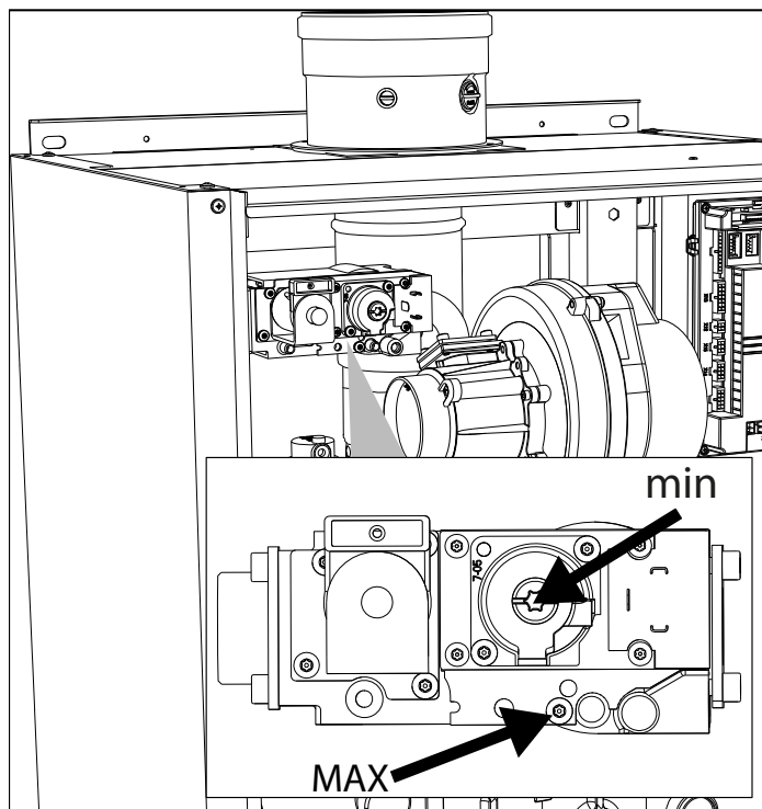
fig. 78- Réglage maxi et mini modèles W 99, W 120 et W 150
