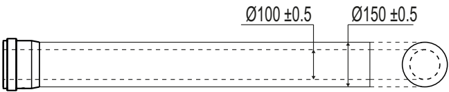
Tolérance des conduits coaxiaux Ø100/150
