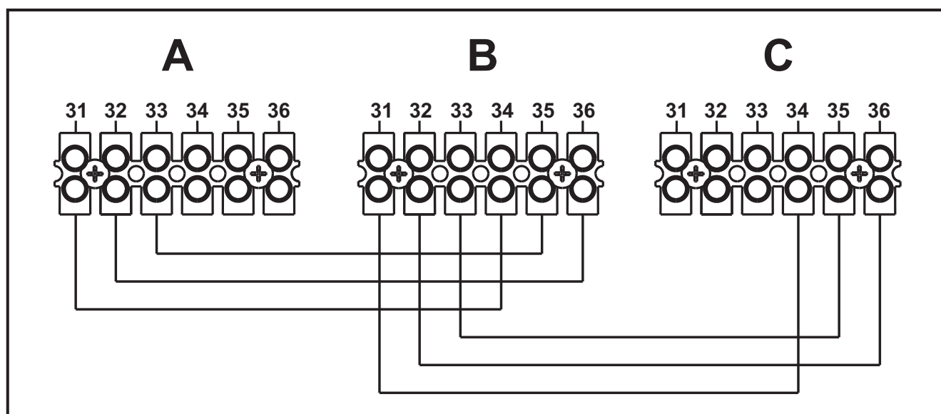
fig. 53 - Conexión en cascada
