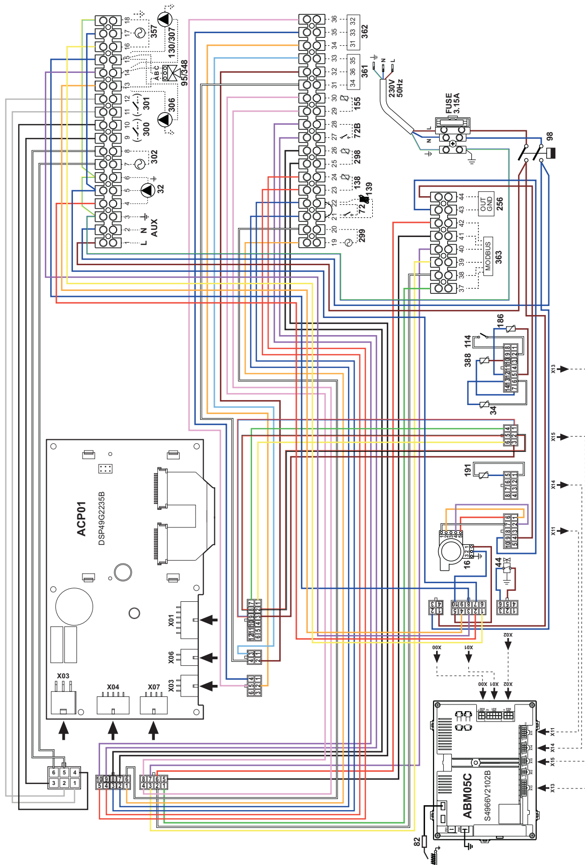
fig. 100- Schéma électrique modèles TORO W 99, TORO W 120 et TORO W 150
