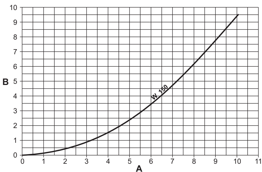
fig. 94- Diagramme perte de charge modèles TORO W 150
