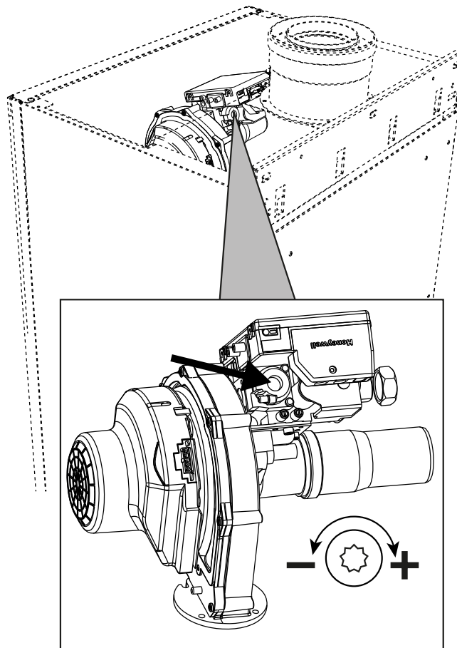
fig. 77- Réglage minimum modèles W 60 et W 80
