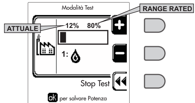
fig. 79 - Modalità TEST (esempio potenza riscaldamento = 80%)
