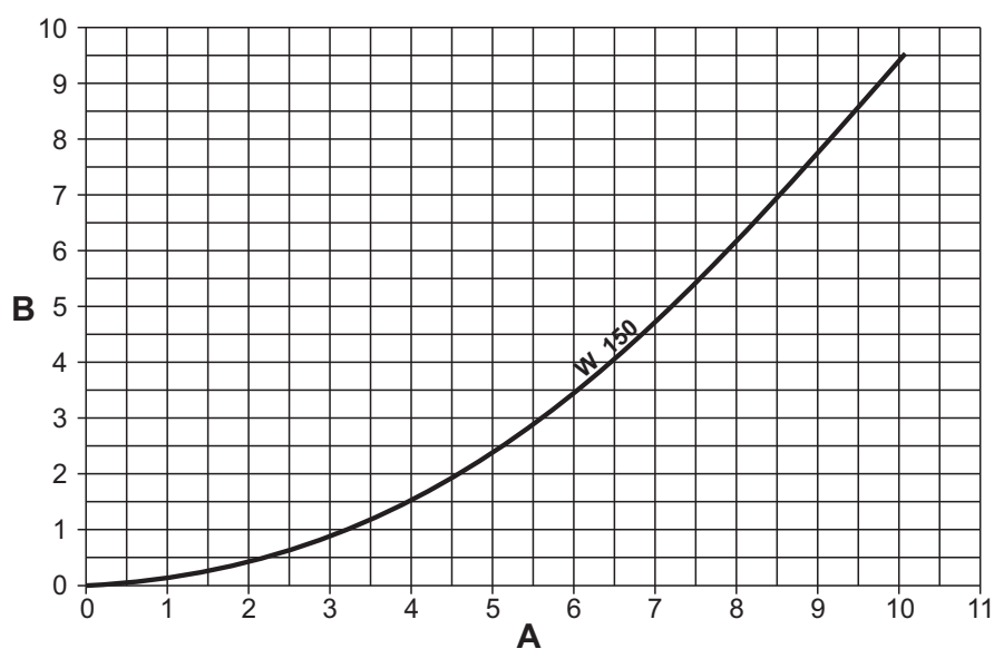
fig. 94- Diagrama de pérdida de carga modelos TORO W 150
