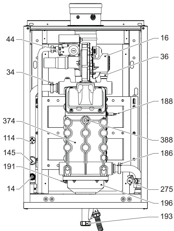
fig. 89- Vista general mods. TORO W 60 y TORO W 80
