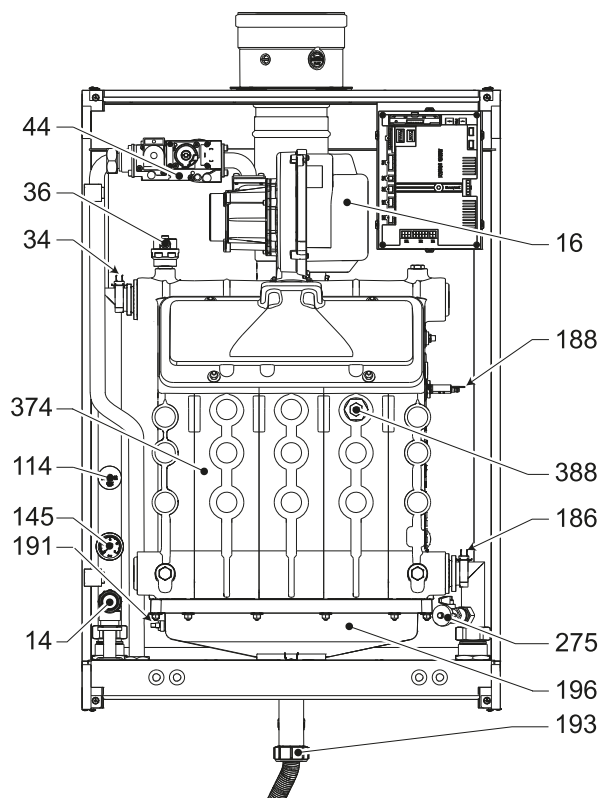
fig. 91- Vista general mod. TORO W 150
