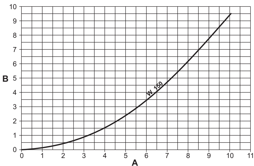
рис. 94- Диаграмма потери нагрузки для моделей TORO W 150
