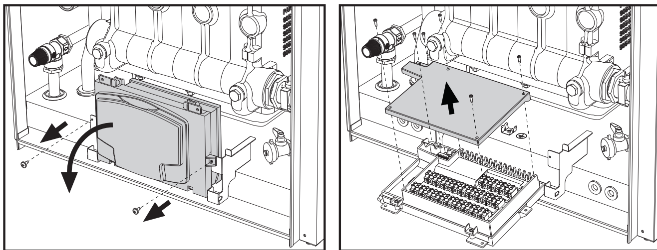
fig. 52 - Morsetteria elettrica
