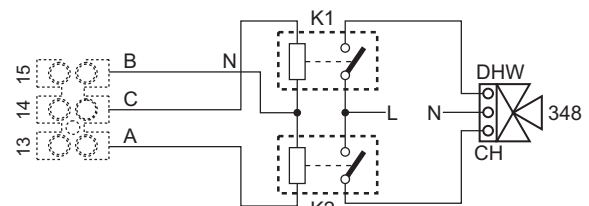
fig. 97- Raccordement de la vanne 3 voies à 3 fils
