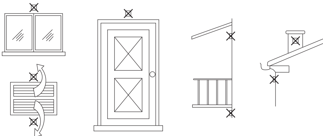
fig. 51- Posición desaconsejada de la sonda exterior
