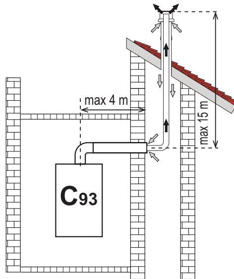
fig. 62 - Esempi di collegamento a canne fumarie (⇨ = Aria / ⇨ = Fumi)
