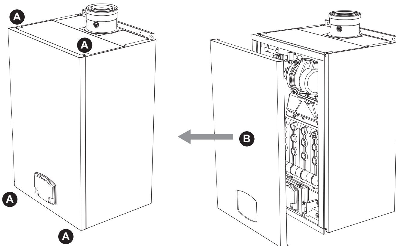
рис. 82- Открытие передней панели
