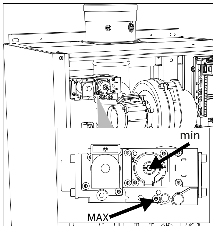
fig. 78- Regulación máxima y mínima modelos W 99, W 120 y W 150
