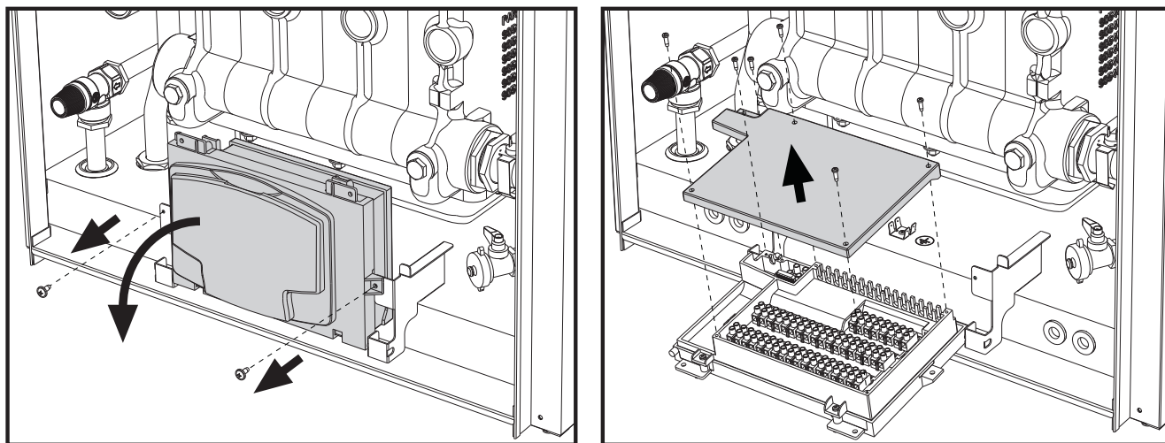
fig. 52- Bornier électrique
