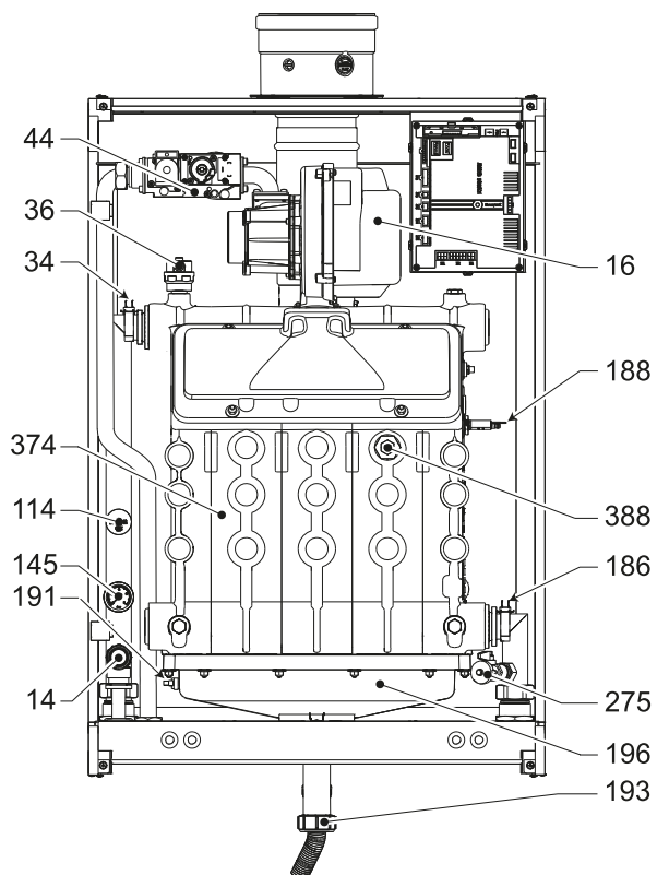
fig. 91- Vue générale mod. TORO W 150
