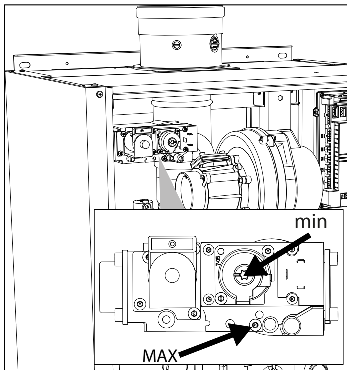
рис. 78- Максимальная и минимальная регулировка моделей W 99, W 120 и W 150
