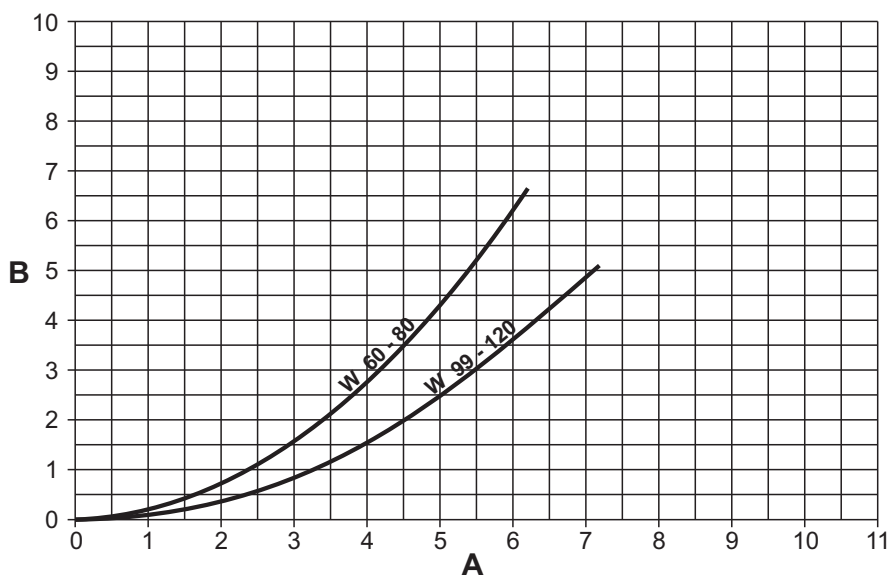
fig. 93- Diagramme perte de charge modèles TORO W 60 - TORO W 80 - TORO W 99 - TORO W 120
