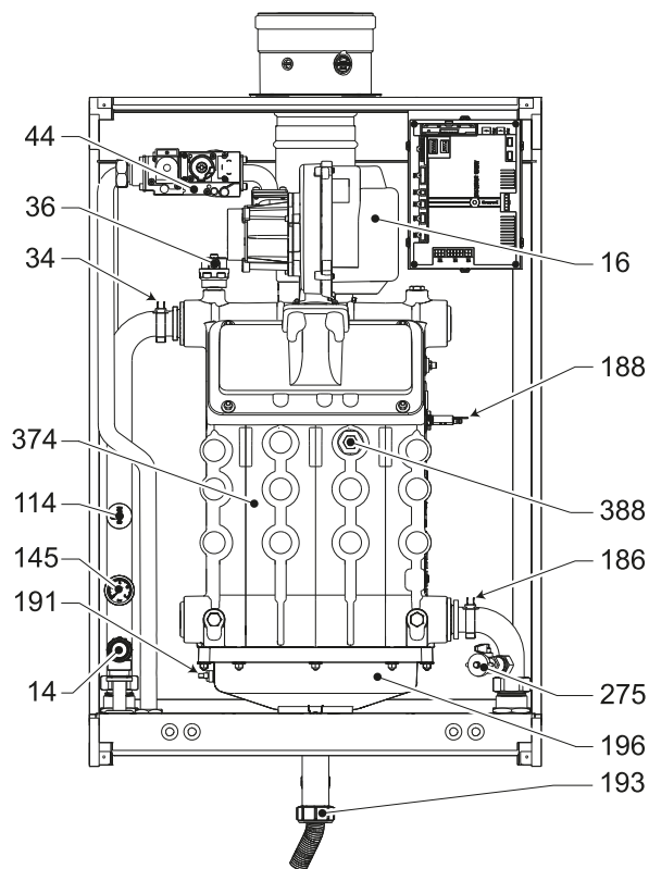
fig. 90- Vue générale mod. TORO W 99 et TORO W 120
