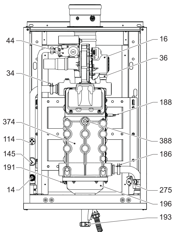
рис. 89- Общий вид, мод. TORO W 60 и TORO W 80
