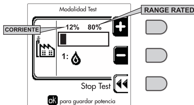
fig. 79- Modo TEST (ejemplo potencia de calefacción = 80%)
