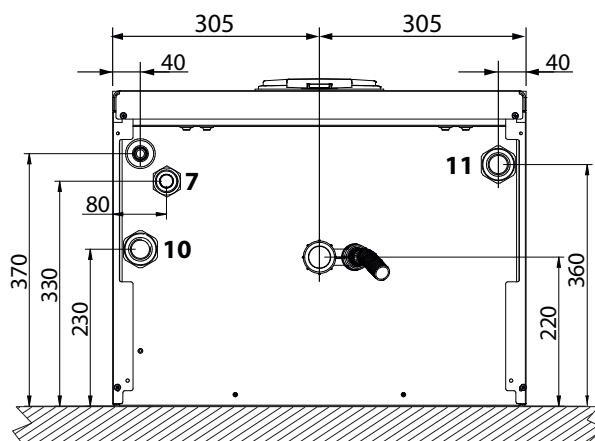
fig. 88- Vue de dessous
