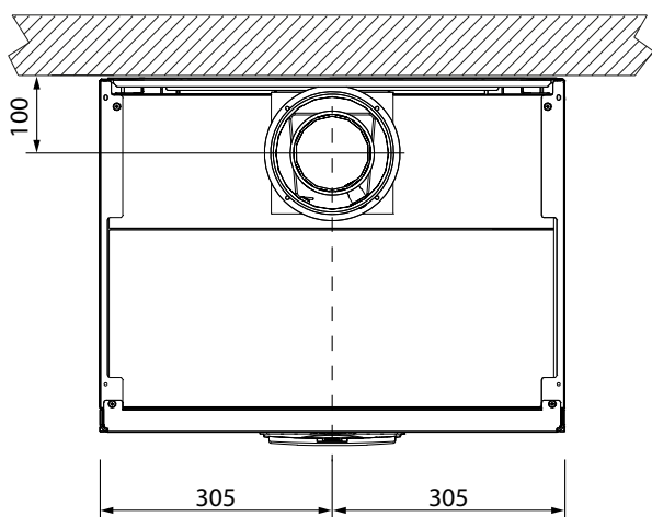
fig. 87- Vue de dessus
