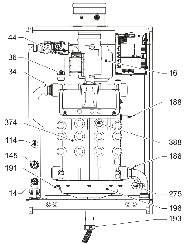
fig. 90- Vista general mods. TORO W 99 y TORO W 120
