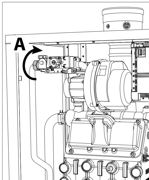
fig. 69 - Modelli W 99, W 120 e W 150
