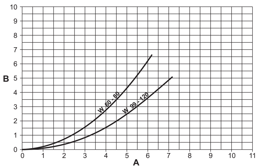
fig. 93- Diagrama de pérdida de carga modelos TORO W 60 - TORO W 80 - TORO W 99 - TORO W 120
