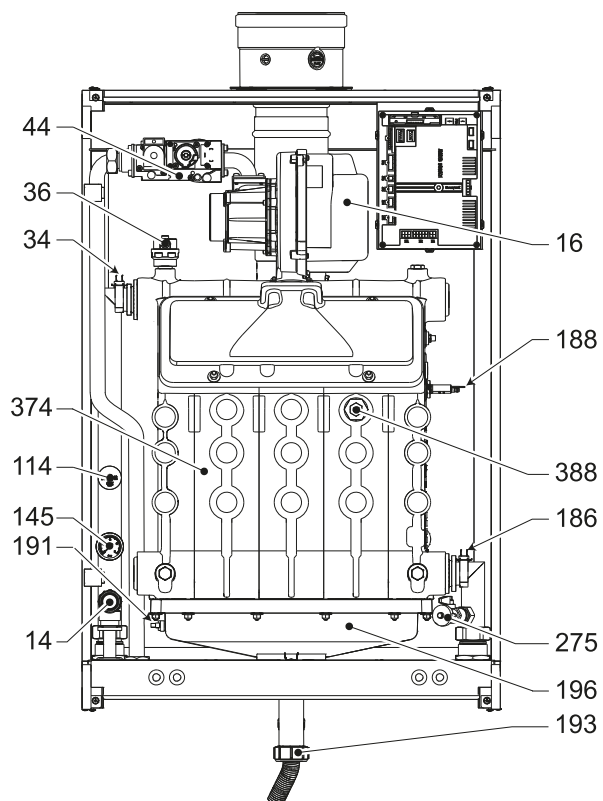
fig. 91 - Vista generale mod. TORO W 150
