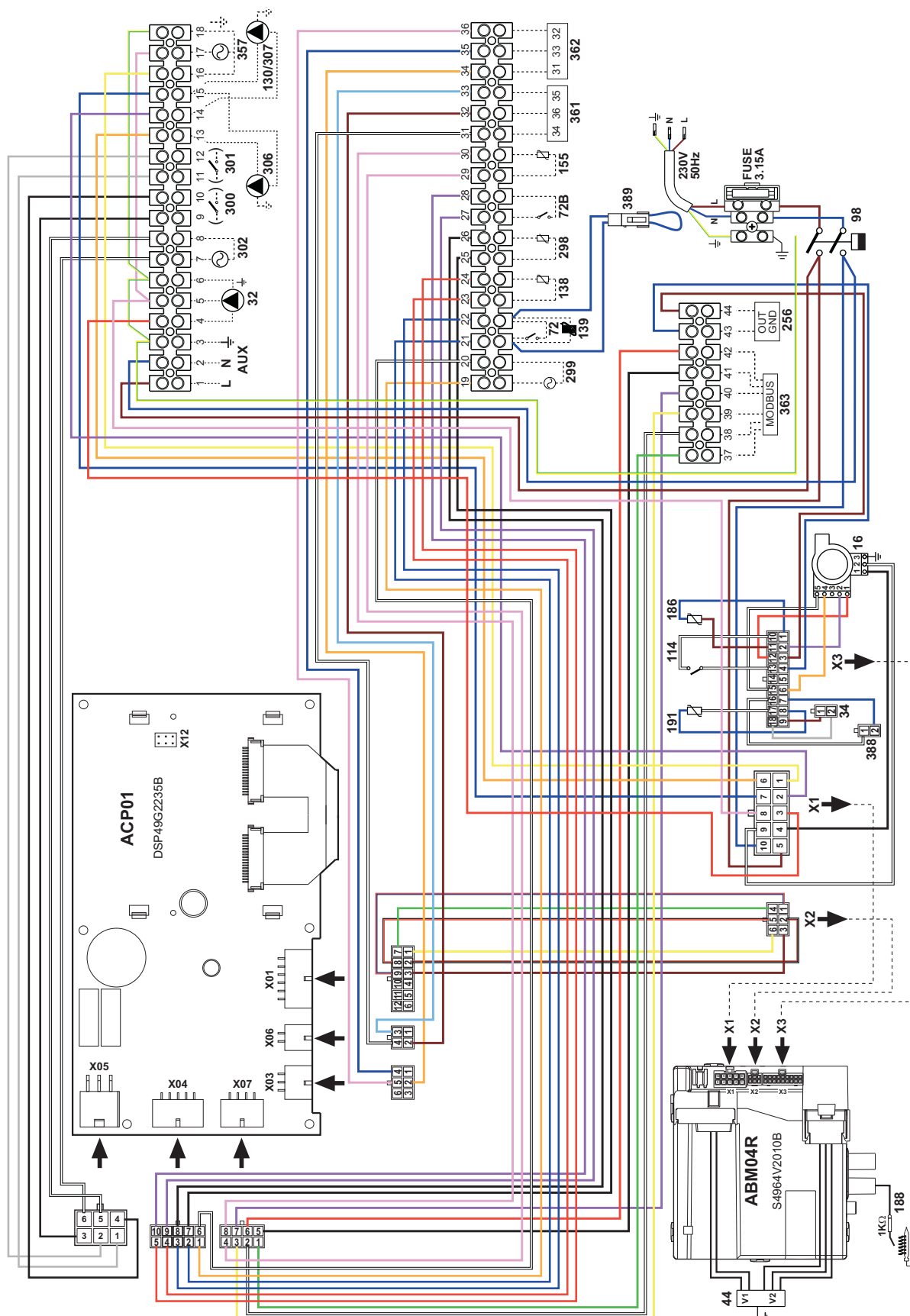
рис. 100- Электрическая схема моделей TORO W 99, TORO W 120 и TORO W 150
