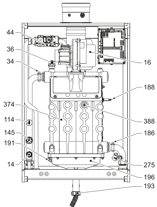
fig. 90 - Vista generale mod. TORO W 99 e TORO W 120
