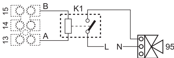
fig. 96- Raccordement de la vanne 3 voies à 2 fils
